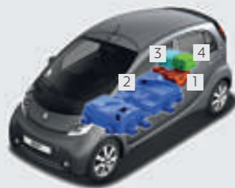
Chaîne de traction électrique 1. Moteur électrique 2. Pack batterie 3. Onduleur 4. Chargeur embarqué
